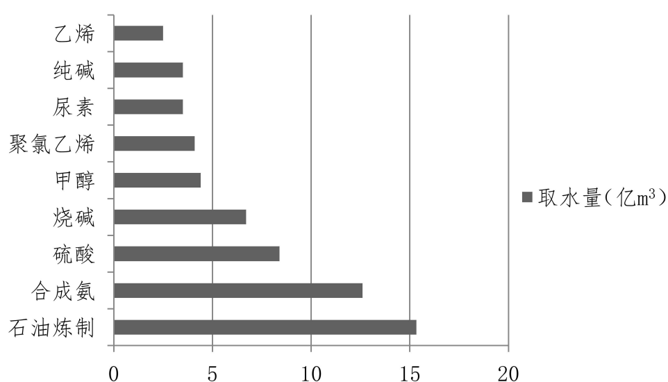
图1 2010年我国石化和化工主要产品取水情况
